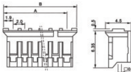
• XJ2006J-A(PH)
