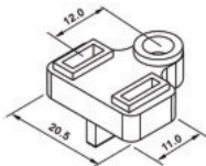
材料(Material): PBT UL94V-0 颜色(Color): 黑色(Black)
