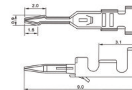
• XJ2008J-Y(SAN)
