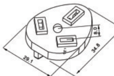
材料(Material): PBT UL94V-0 颜色(Color): 黑色(Black)
