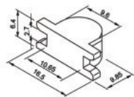
材料(Material): PBT UL94V-0 颜色(Color): 黑色(Black)
