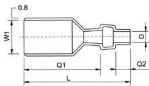
250直形护套
