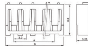
• XJ2008J-Y(SAN)
