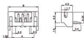
• XJ2006J-QA(PH)
