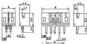
• XJ2006J-QA(PH)
